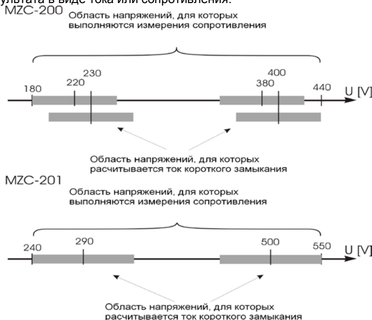
Рис. 9. Зависимости между напряжением сети и возможностью вычисления ожидаемого тока короткого замыкания на примере MZC-200 и MZC-201
