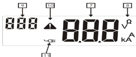
Рис.2. Дисплей измерителей семейства MZC-200
