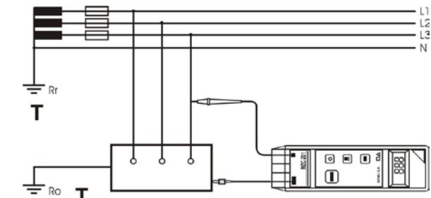
Рис. 8б. Тестирование эффективности защиты корпуса электроустановки сети T-T
