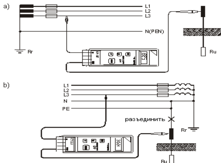
Рис. 10. Способ подключения измерителя семейства MZC-200 при измерениях сопротивления заземления
