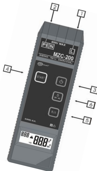
Рис.1. Расположение гнезд и клавиш в измерителях семейства MZC-200 (лицевая панель)
