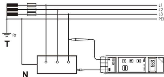
Рис. 8а. Тестирование эффективности защиты корпуса электроустановки сети T-N
