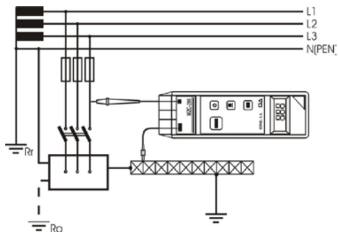
Рис. 11. Контроль целостности нулевых защитных проводников и уравнивательных соединений.
