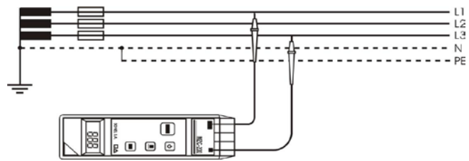
Рис.7. Измерение в рабочей цепи (L-L)
