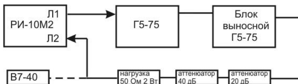
Рисунок 9-8 Схема определения чувствительности приёмного тракта
