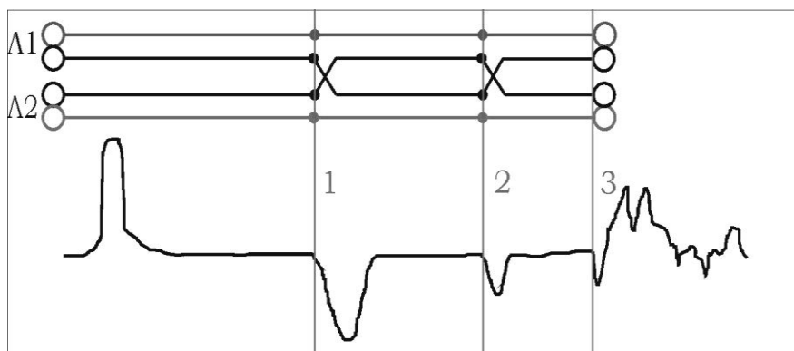
Рисунок 6-8 «Разбитость пар»
