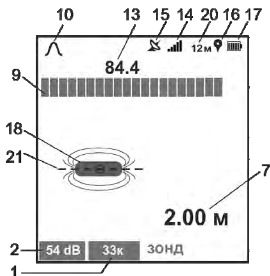
Рисунок 3.4 – Индикация приемника в режиме «ЗОНД»
