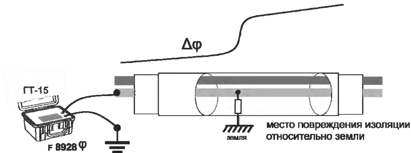
Рисунок 5.3.3.2 – Схема подключения и сдвиг фазы при поиске повреждения изоляции фазовым методом
