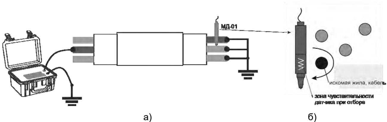
Рисунок 5.4.1 – Схема подключения при отборе жил кабеля
