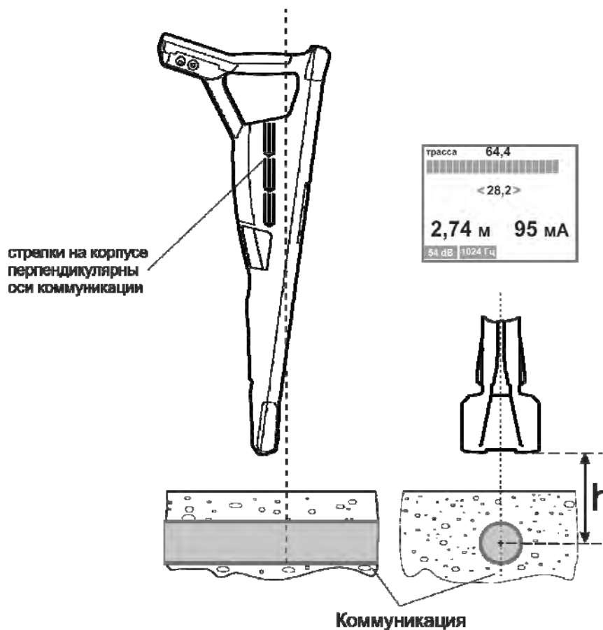
Рисунок 4.3 – Показания глубины залегания и тока
