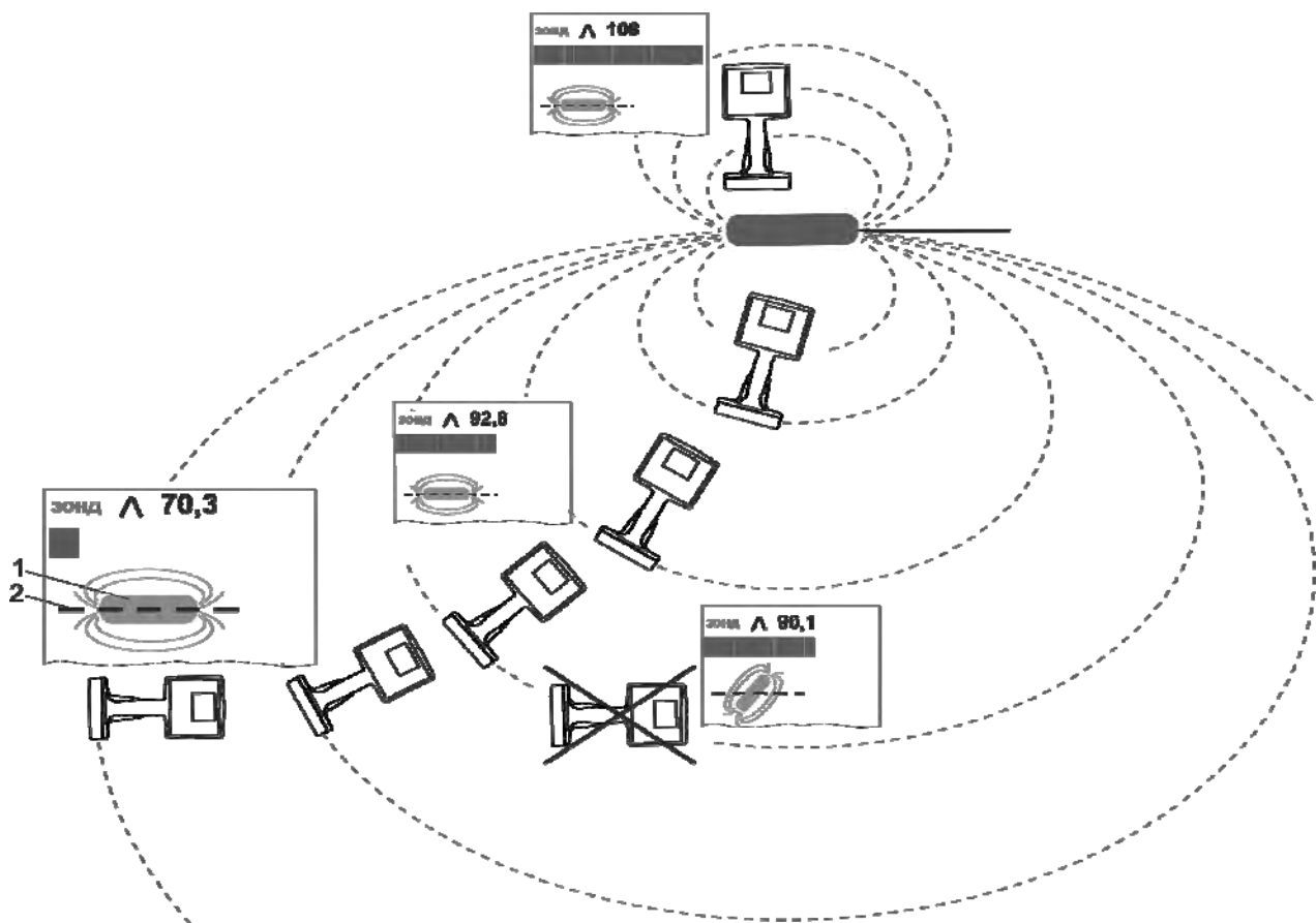
Рисунок 4.5.1 – Поиск местоположения зонда
