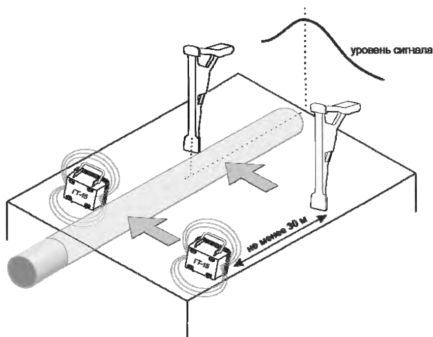
Рисунок 4.4.2 б – Обследование участков местности с помощью ГТ-15
