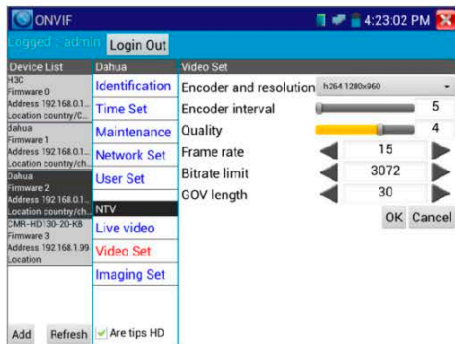
Рис.3.3.3-8 Установка разрешения воспроизведения
