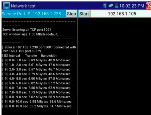
Рис. 3.3.24-4 Запуск сервера
