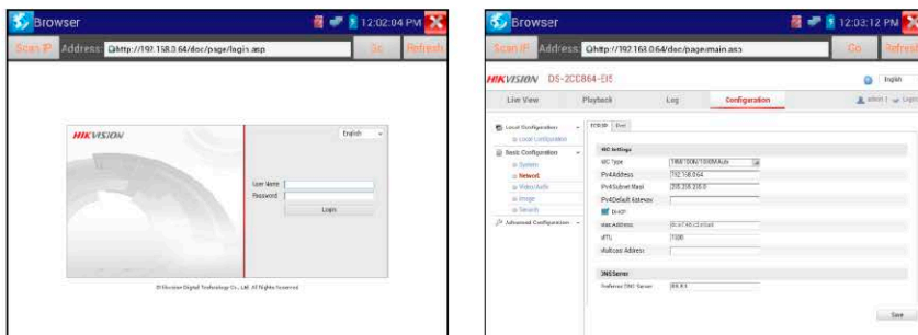
Рис.3.3.21-1 Встроенный браузер
