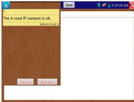
Рис.3.3.24-8 Блокнот
