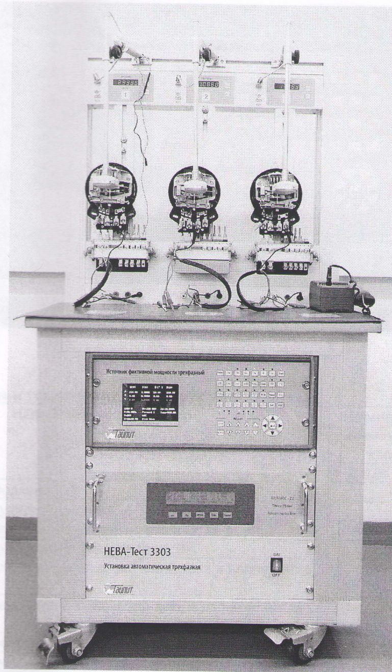
Рис.1 Установка НЕВА-Тест 3303Л
