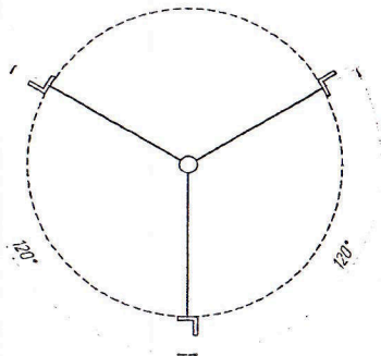
Рисунок 1 – Схема размещения растяжек в плане
