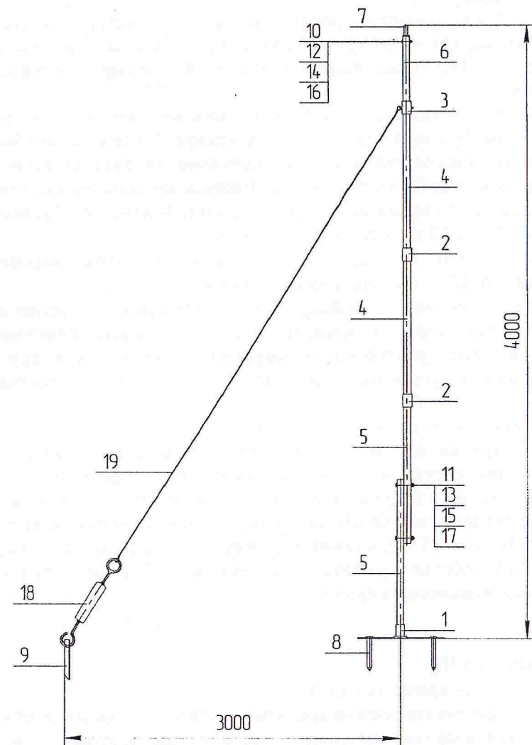
1 – основание; 2 – втулка; 3 – втулка; 4 – стойка; 5 – стойка; 6 – стойка; 7 – штырь; 8 – штырь; 9 – штырь; 10 – болт; 11 – болт; 12 – гайка; 13 – гайка; 14 – шайба; 15 – шайба; 16 – шайба; 17 – шайба; 18 – талреп; 19 – растяжка
