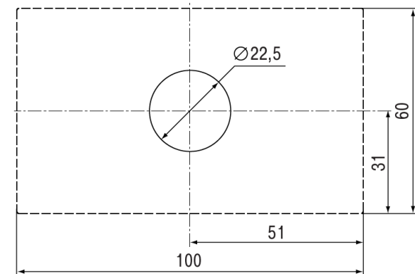
Рисунок 2.2 – Установочные размеры прибора
