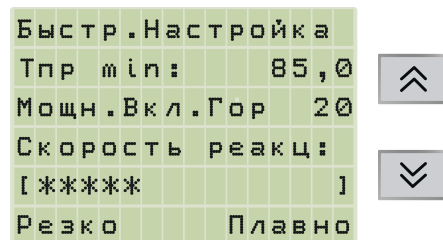
Рисунок 6.9 – Меню «Быстрая настройка» для каскадных регуляторов
