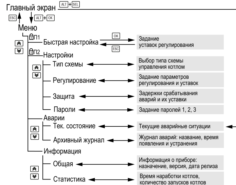
Рисунок 6.1 – Схема переходов по меню ИПП120 для КТР-121.01.10
