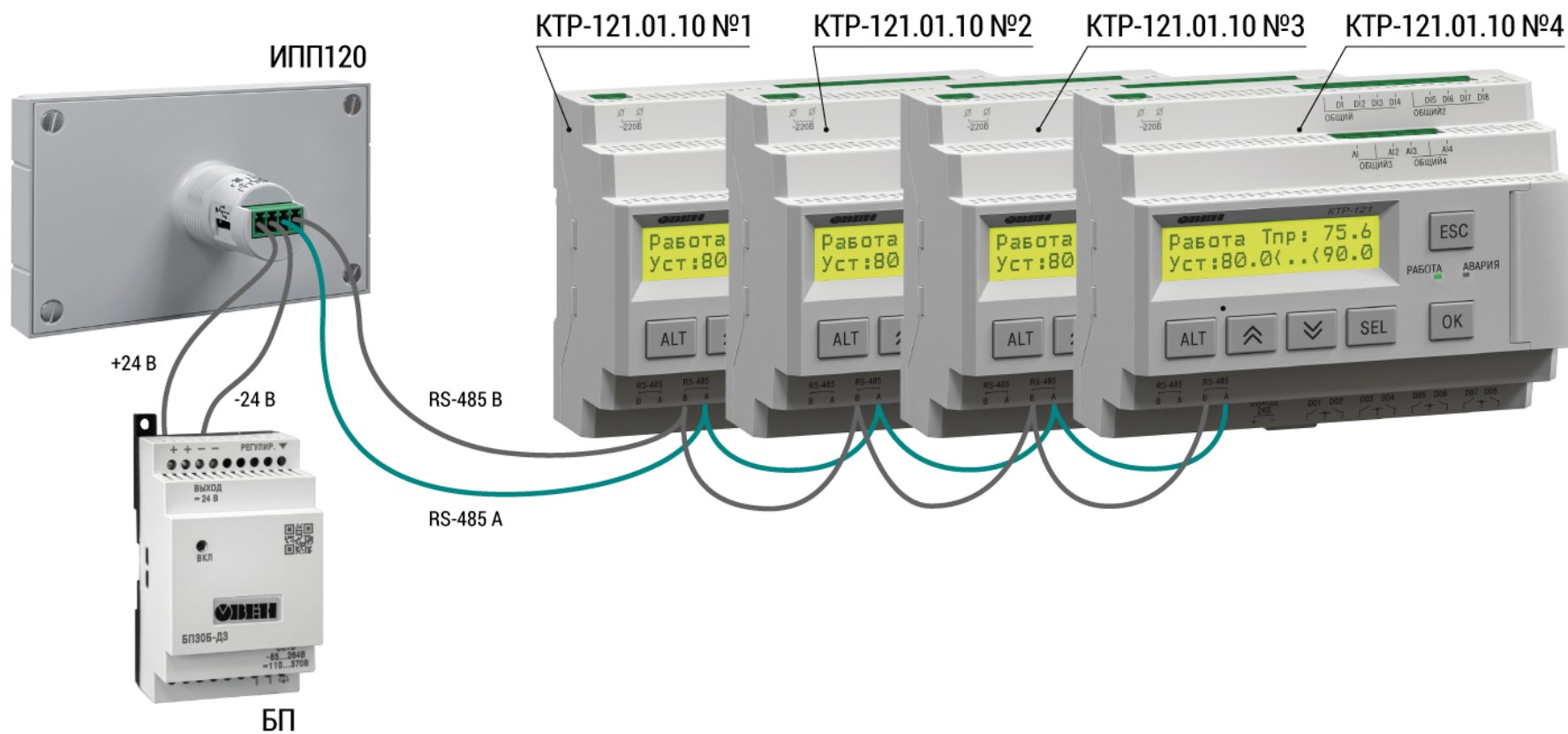
Рисунок 3.4 – Пример схемы подключения связки ИПП120 + 4 × КТР-121.01.10
