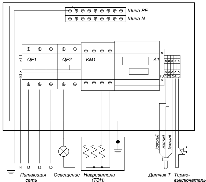
Схема подключения блоков типа БУК-1-3-6.0; БУК-1-3-9.0; БУК-1-3-12.0.
