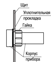
Рисунок 1 – Монтаж прибора щитового крепления
