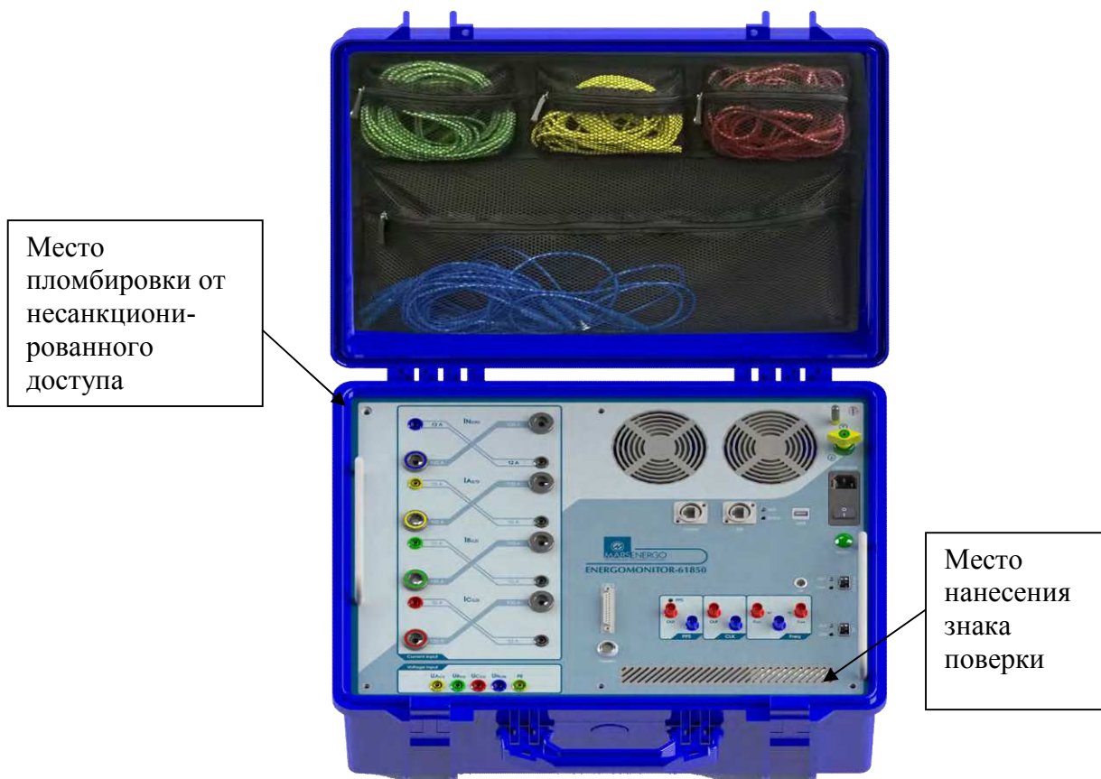
Рисунок 1 - Общий вид модификации "Энергомонитор-61850 II", место пломбировки от несанкционированного доступа и обозначение места нанесения знака поверки
