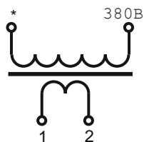
Рис. 2 Схема соединения обмоток
