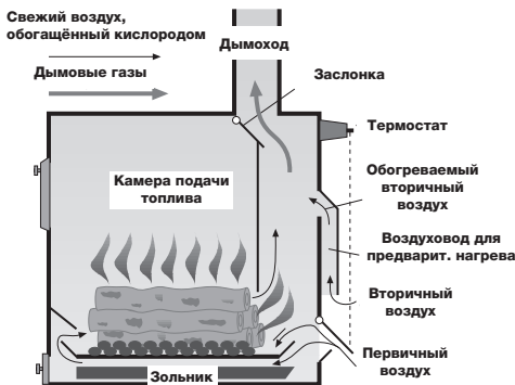
Рис. 6: Простая колосниковая печь
