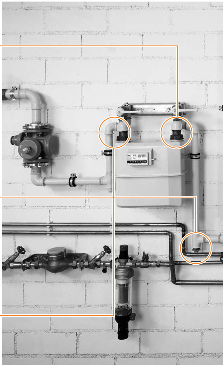
Проведение предварительного теста с использованием прибора testo 312-3
