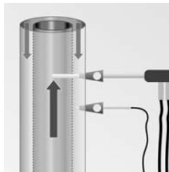
Рис. 9: Измерение температуры в дымоходе
