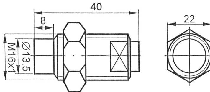
Рис. 2в. Общий вид чувствительного элемента датчика оборотов ВК-317.01.
