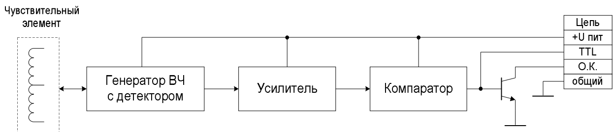
Рис. 4. Структурная схема датчиков оборотов.
