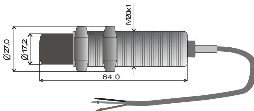
Рис. 2а. Общий вид датчика оборотов ВК-317
