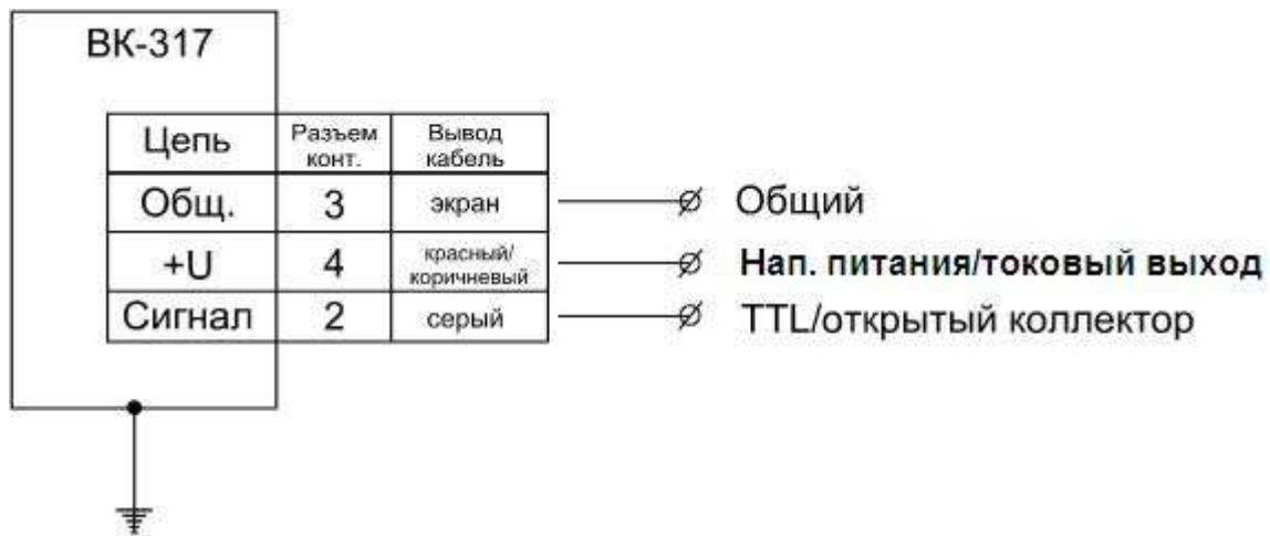
Рис. 13. Назначение контактов разъема или кабельных выводов датчиков оборотов ВК-317 и ВК-317-1 (цвет проводов указан для поставки датчика оборотов с кабельными выводами). Назначение контактов клеммной колодки датчика оборотов ВК-317.01 указано на корпусе согласующего усилителя.
