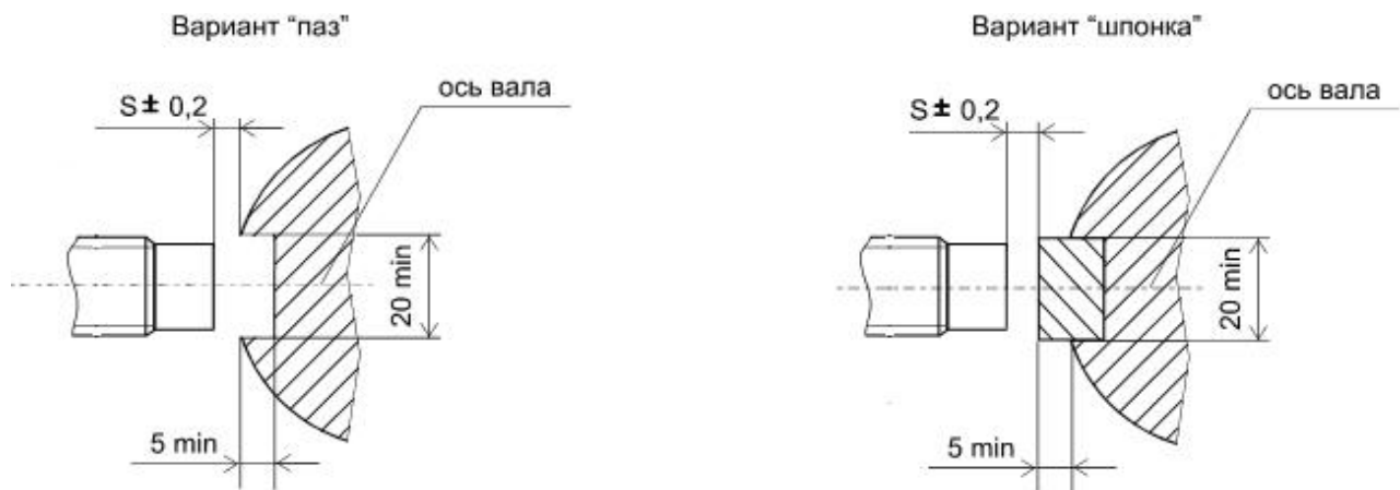
Рис. 5. Установка датчиков оборотов (чувствительного элемента датчика).
