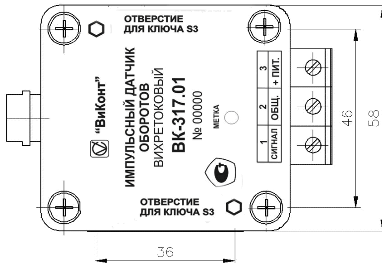
Рис. 3. Общий вид согласующего усилителя датчика оборотов ВК-317.01.
