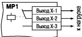
Рисунок Б.2 – Схема подключения к выходному устройству типа P (электромагнитное реле)
