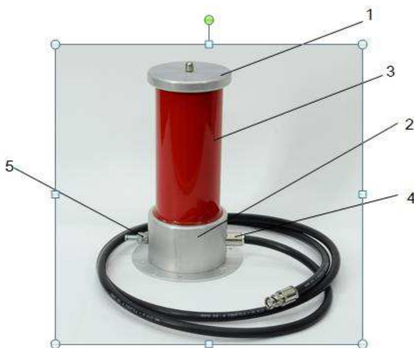
1 - высоковольтный электрод; 2 - основание; 3 - диэлектрический цилиндр; 4 - гнездо приборное; 5 - зажим защитного заземления.
