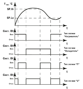
Рисунок 8.1 – Типы логики работы прибора
