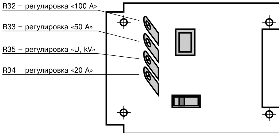
Рис. 3. Расположение регулировочных элементов на плате прибора «Квант»
