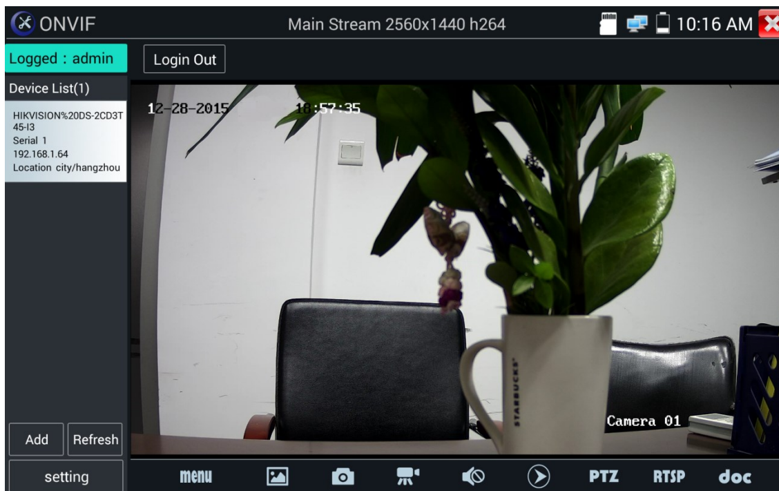
Рис.8 Настройка ONVIF
