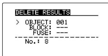
Рисунок 6.8: Меню стирания измерений (выбрана область структуры данных)
