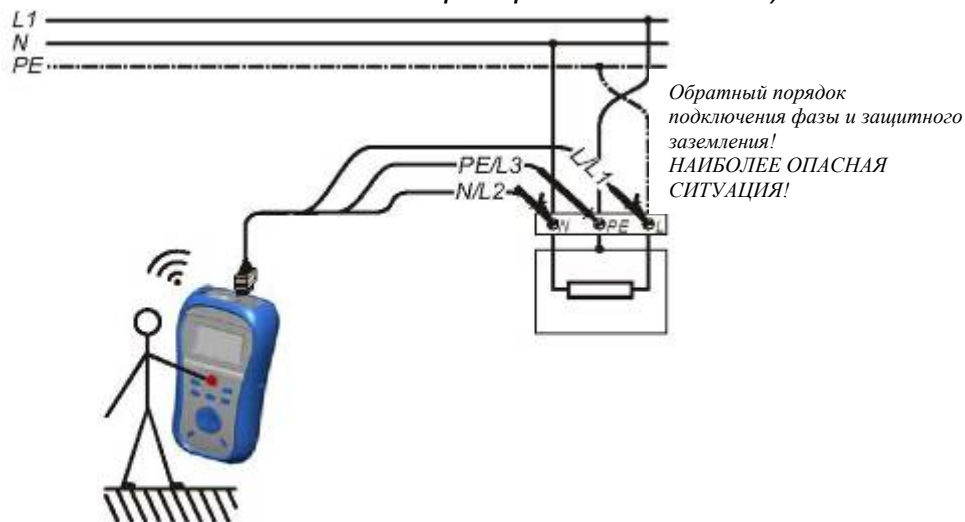
Рисунок 5.18: Поменянные местами проводники L (фаза) и PE (ЗЗ) (применение кабеля проверки подключения)
