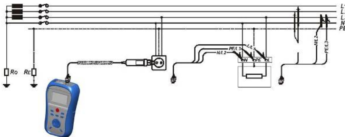
Рисунок 5.12: Измерение полного сопротивления линии фаза-нейтраль или фаза-фаза – подключение управляющего кабеля и универсального тестового кабеля
