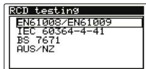
Рисунок 4.6: Выбор стандарта тестирования УЗО
